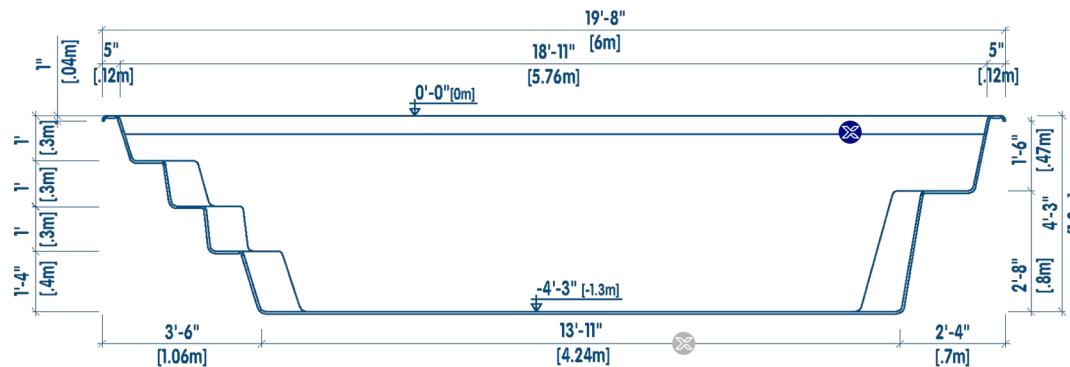
CORTE LONGITUDINAL | LONGITUDINAL SECTION
